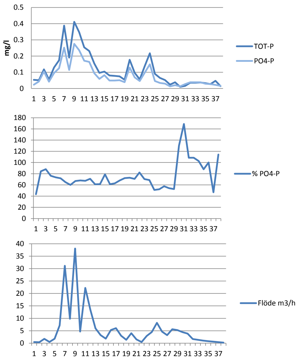
Figur 13 (övre): Koncentrationerna för totalfosfor (TOT-P) och fosfatfosfor (PO4-P) i Lagga under mätperioden 30 okt 2009 till 8 maj 2011. (mellan): andelen fosfatfosfor av totalfosfor under samma period. Koncentrationen fosfatfosfor är vid några tillfällen med låga koncentrationer högre än totalfosfor, vilket visar på osäkerheterna i fosfatfosforanalyser vid låga koncentrationer. (nedre): Vattenflödet genom dammen i m³/h vid mättillfällena. X-axeln visar antalet mättillfällen för vilka proverna skickats till laboratorium för analys.
