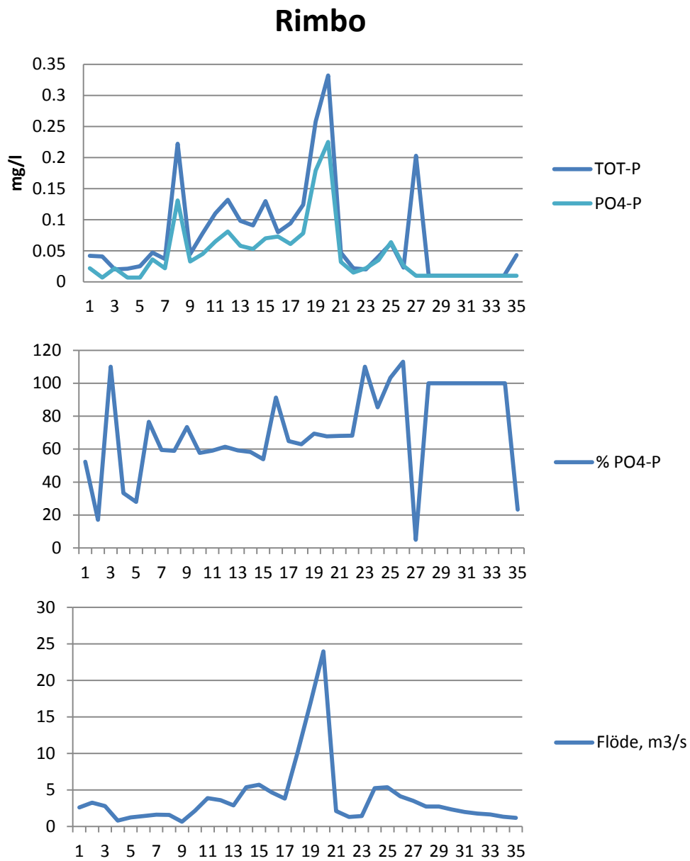
Figur 14 (övre): Koncentrationerna för totalfosfor (TOT-P) och fosfatfosfor (PO4-P) i Rimbo under mätperioden 1 december 2009 till 20 april 2011. (mellersta): andelen fosfatfosfor av totalfosfor under samma period. (nedre): Vattenflödet genom sidodammen i m 3 /h vid mättillfällena. X-axeln visar antalet mättillfällen för vilka proverna skickats till laboratorium för analys.
