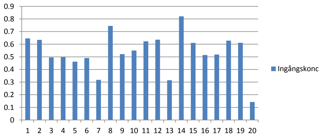
Figur 20. Reningsgrad, uppehållstid och ingångskoncentration för Väringe. Hela mätperioden från 7 oktober 2010 till 24 april 2011. Anläggningen var i drift från augusti 2010 men diket låg torrt till början av oktober, och även efter den 24 april våren 2011.
