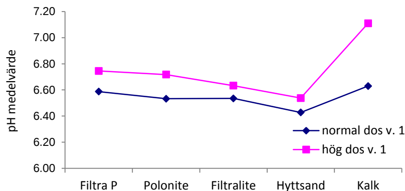
Figur 26. pH-värdet i krukor som hade filter/kalktillsats i jorden en vecka efter sådd. Skillnader i pH kunde tillskrivas filter/kalktillsatsen ( p<0,001 ) och dosen ( p<0,001 ). En dag före skörd hade skillnaderna mellan enskilda filter jämnats ut och påverkade inte längre pH signifikant.
