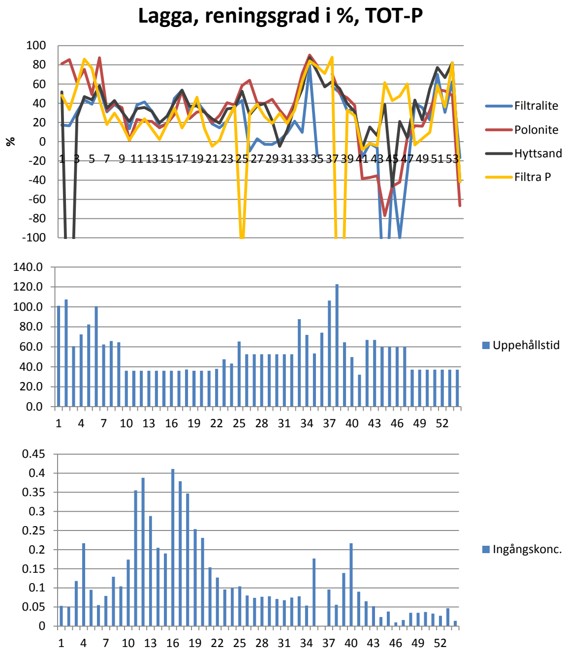
Figur 18. Reningsgrad, uppehållstid och ingångskoncentration för Lagga. Hela mätperioden från 30 oktober 2009 till 8 maj 2011.
