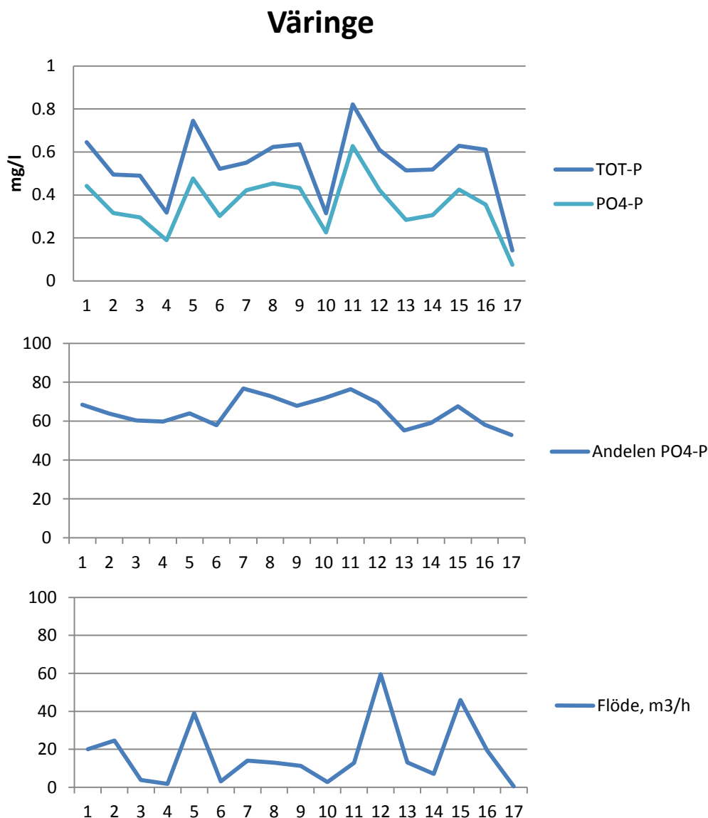
Figur 15 (övre): Koncentrationerna för totalfosfor (TOT-P) och fosfatfosfor (PO4-P) i Väringe under mätperioden 7 oktober 2010 till 24 april 2011. (nedre): andelen fosfatfosfor av totalfosfor under samma period. (nedre): Vattenflödet genom diket i m³/h vid mätillfällena (i Väringe finns ingen sidodamm). X-axeln visar antalet mätillfällen för vilka proverna skickats till laboratorium för analys.
