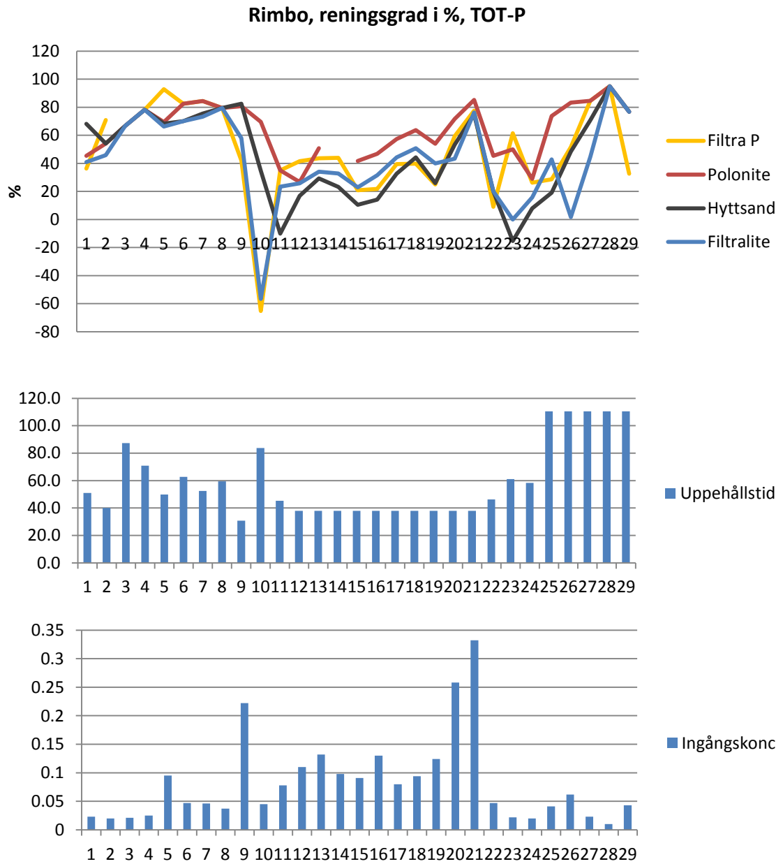
Figur 19. Reningsgrad, uppehållstid och ingångskoncentration för Rimbo. Hela mätperioden från 2 December 2009 till 24 april 2011.
