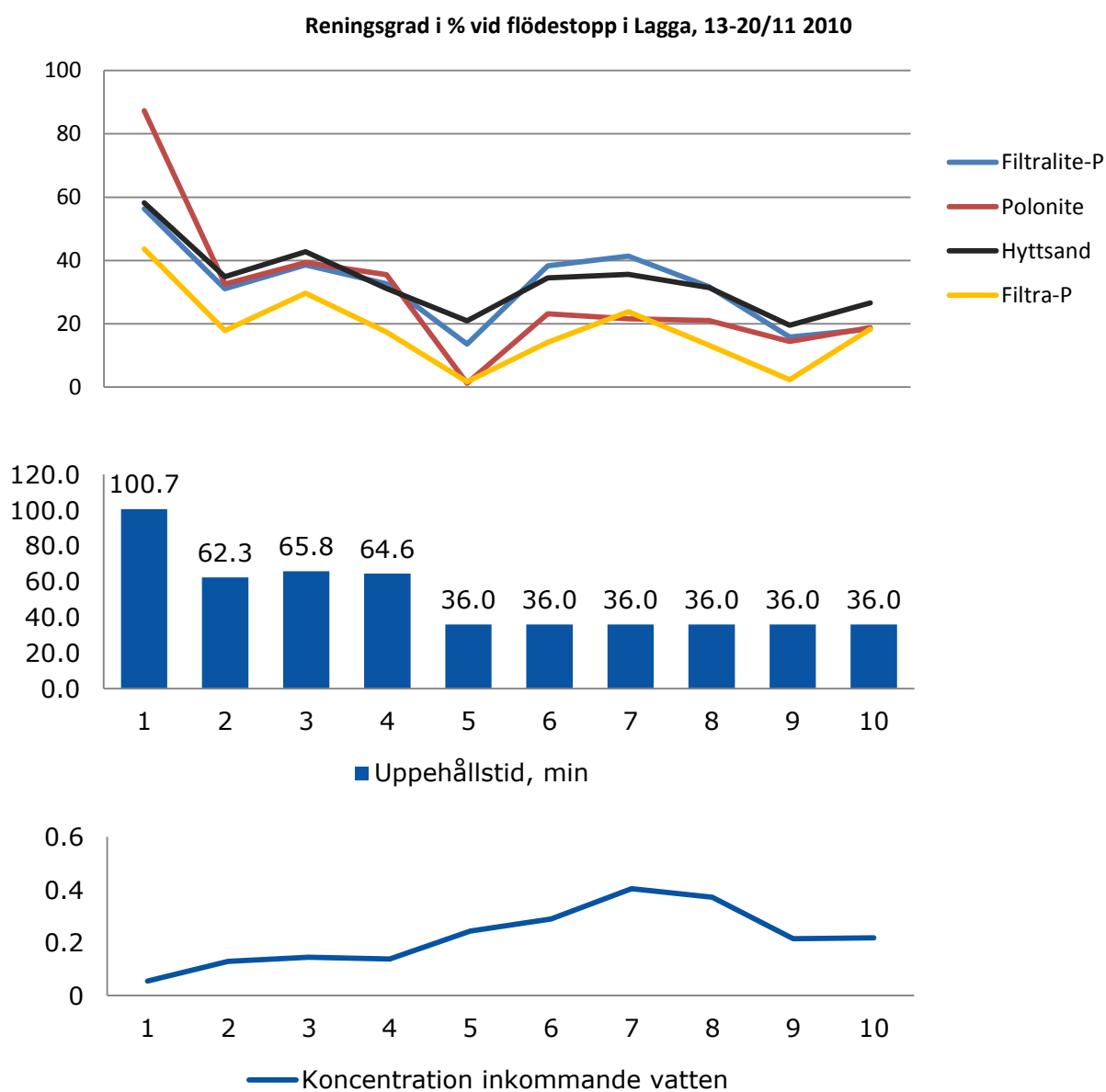
Figur 22. Reningsgrad, uppehållstid och ingångskoncentration TOT-P vid en flödestopp i Lagga.
