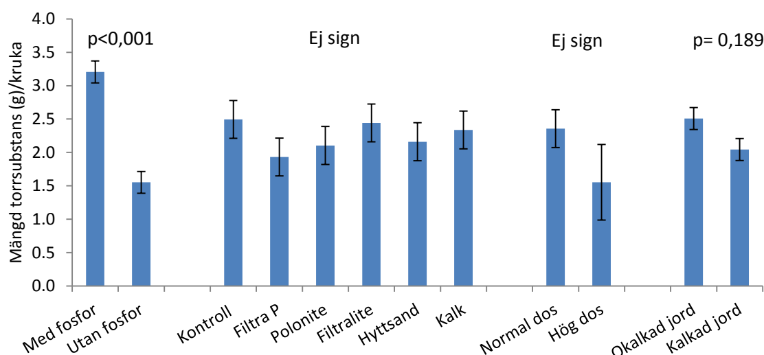
Figur 25. Mängd torrsubstans korn som producerats per kruka. P-värden för betydelse av fosfor, filter/kalk, dos, och jord presenteras ovanför respektive staplar. P-värden < 0,2 redovisas i figuren men endast p < 0,05 betraktas som signifikant.
